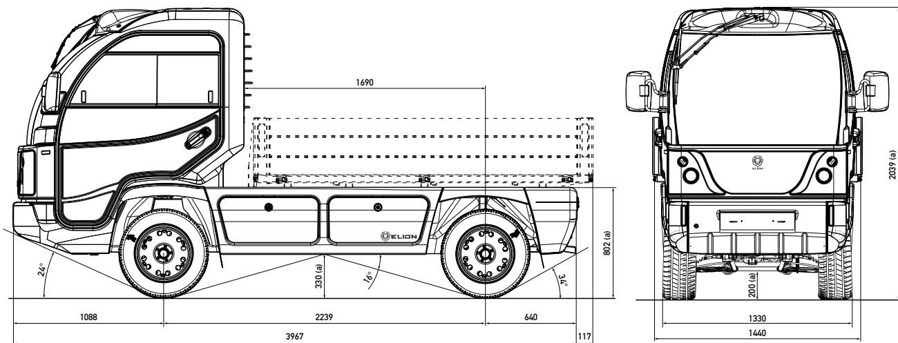
(a) Unbeladenes Fahrzeug
